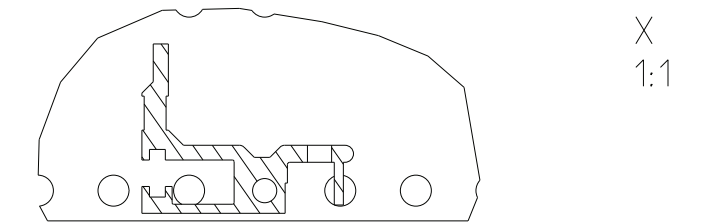
Ausführung 2: Hintere Verbindungsschienen für Einzelsteckverbinder
